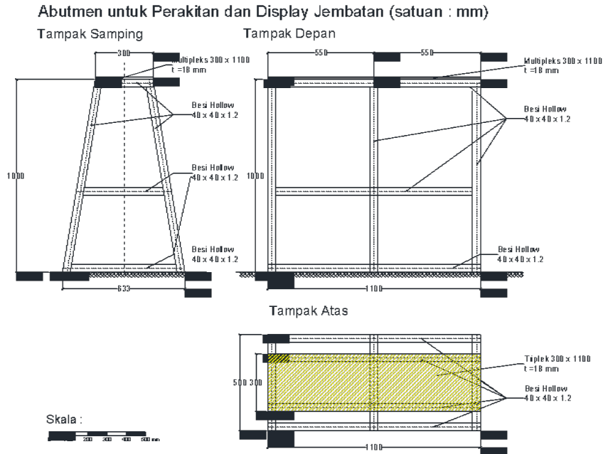
Gambar 10. Abutmen untuk display Jembatan
