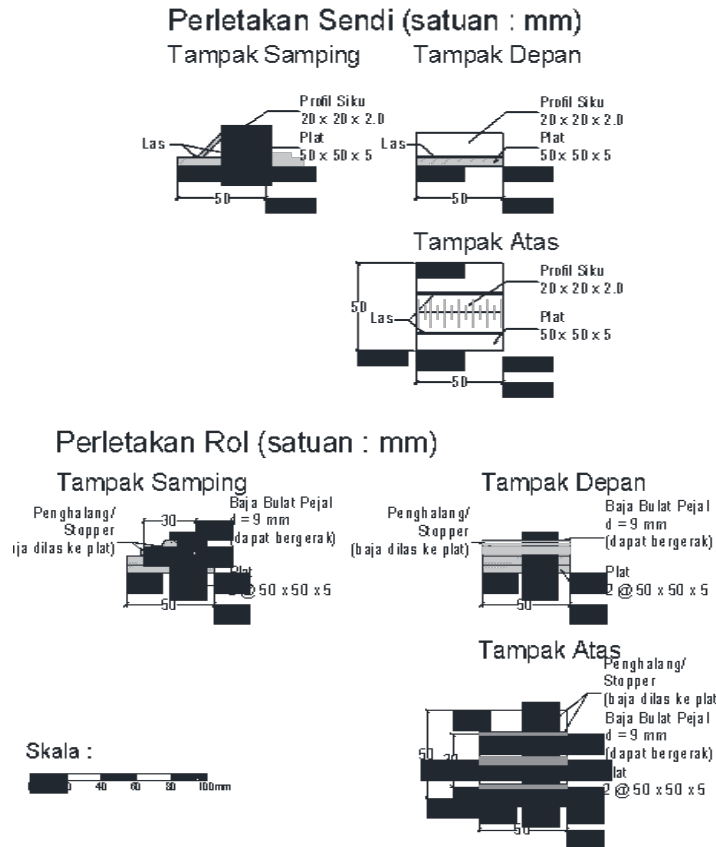
Gambar 25. Tumpuan Rol dan Sendi
