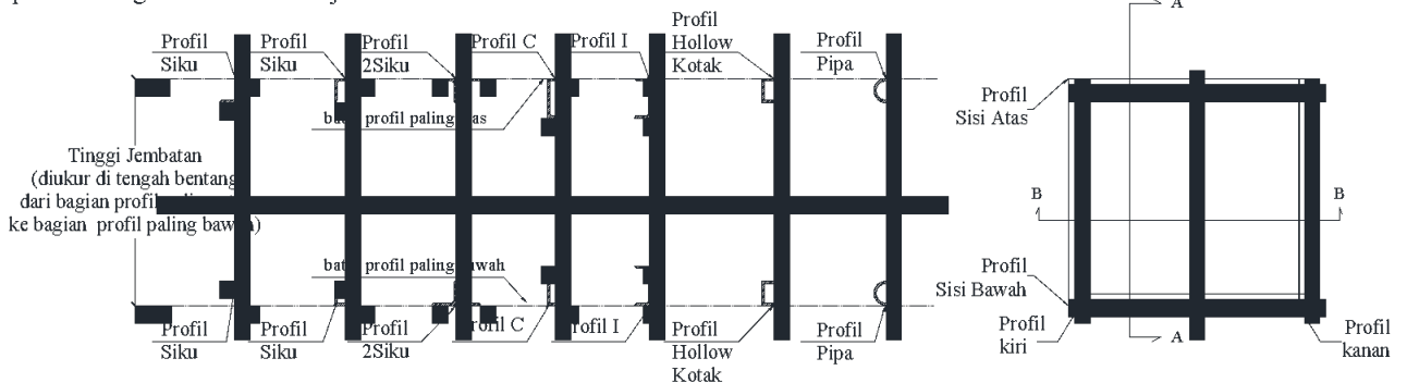
Gambar 13 Contoh Pengukuran Tinggi Jembatan Pada Berbagai Jenis Profil Baja (tambahan)
