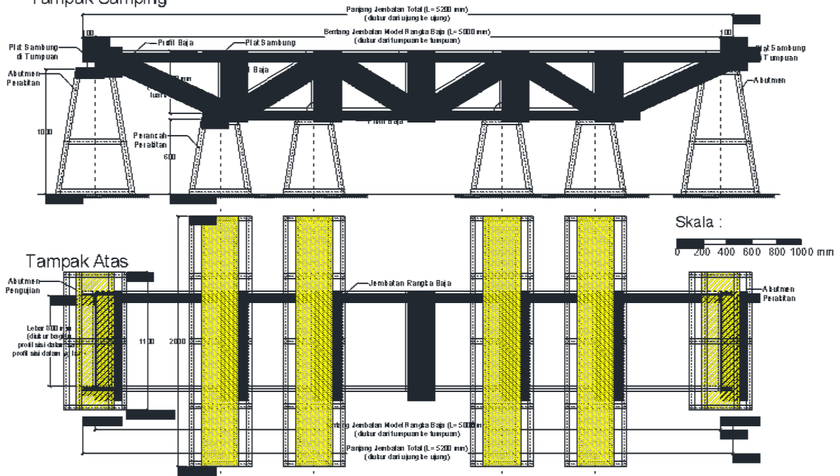
Gambar 2 Perakitan Jembatan Rangka Baja
