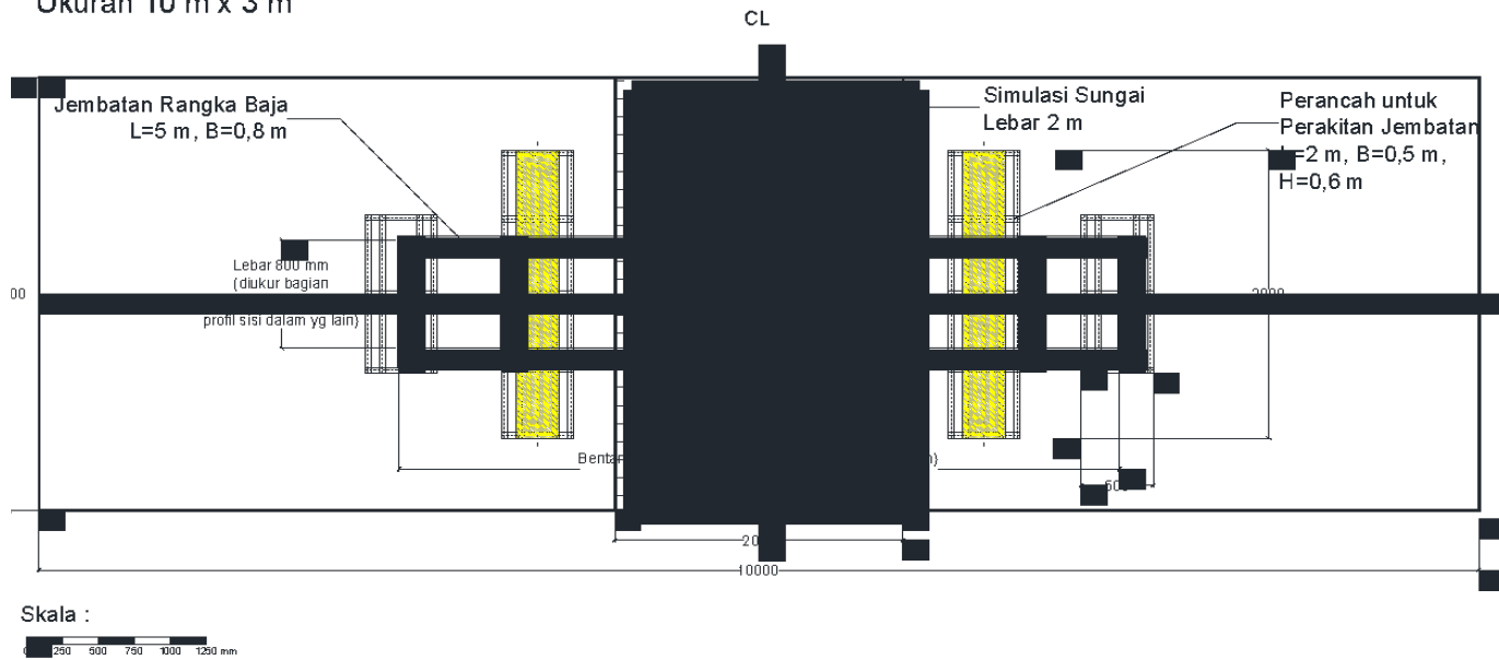
Gambar 4. Site Plan Tempat Perakitan Jembatan Rangka Baja
