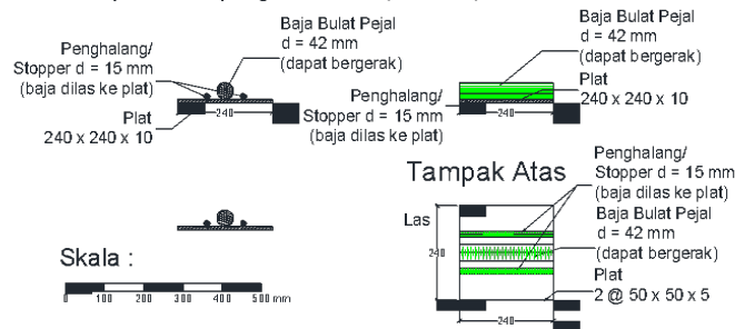
Gambar 11. Tumpuan Rol dan Sendi
