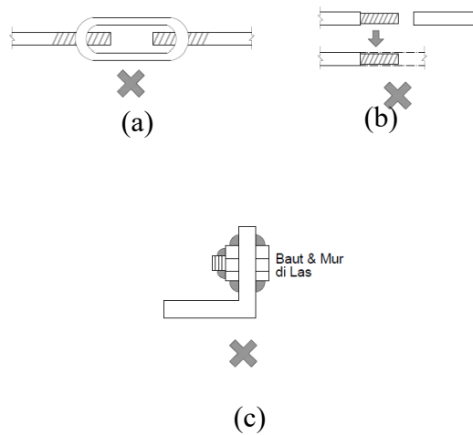
Gambar 5. Sambungan Antar Member Yang Tidak Diijinkan
