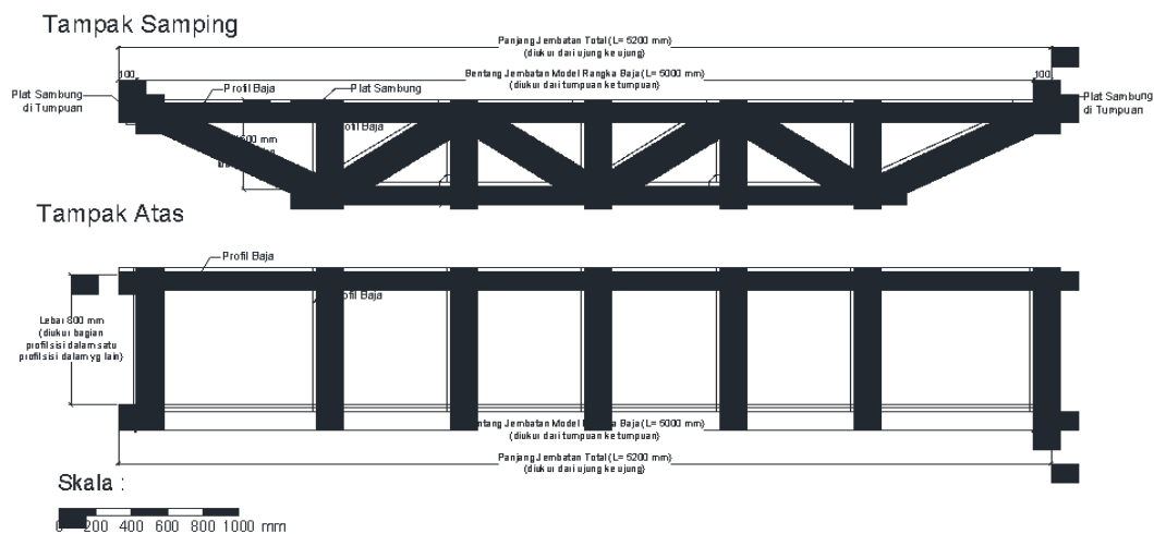
Gambar 1. Bentuk Umum Jembatan Rangka Baja
