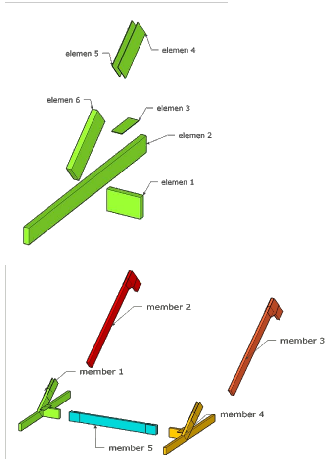
Gambar 18. Sambungan Antar Member Yang Tidak Diijinkan
