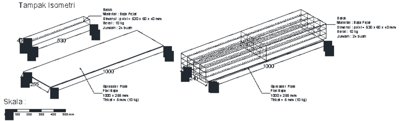
Gambar 27. Beban 250 kg Untuk Pengujian Jembatan Model Pelengkung
