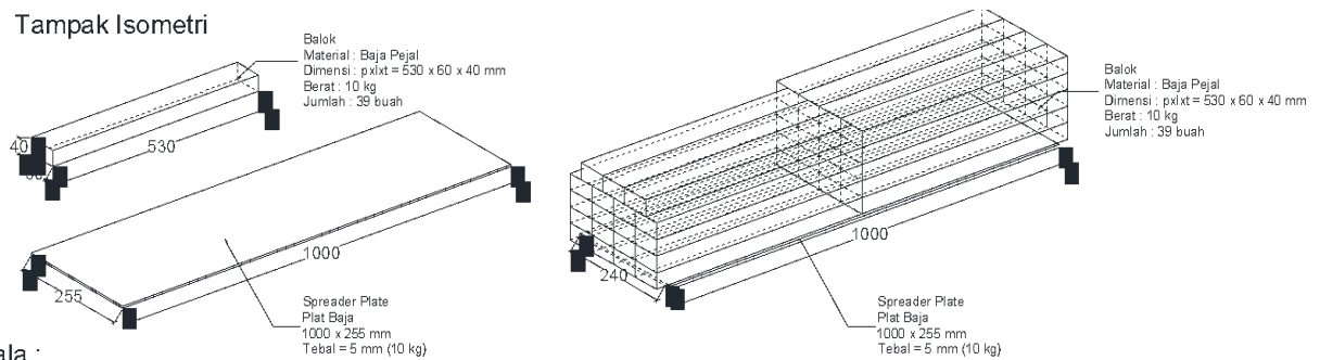
Gambar 12. Beban 400 kg Untuk Pengujian Jembatan Rangka Baja
