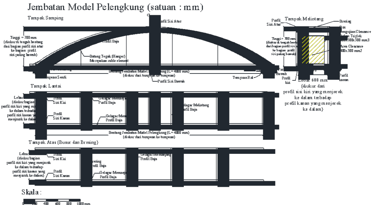
Gambar 15. Bentuk Umum Model Jembatan Pelengkung Tied Arch dan Penempatan Boks Uji Clearance
