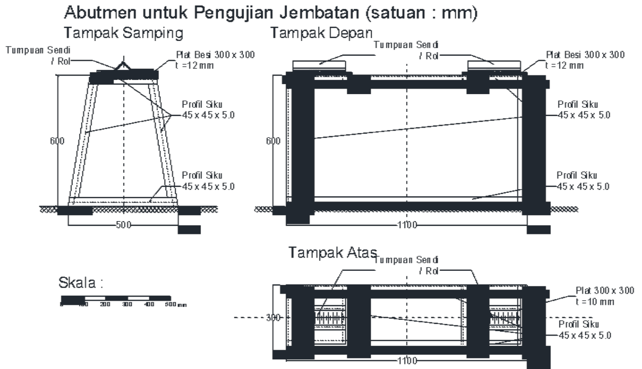
Gambar 20. Abutmen untuk Pengujian Jembatan Boks Pengujian Member (satuan : mm)
