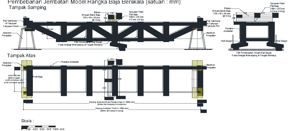
Gambar 3 Penempatan Beban dan Dial pada Jembatan Rangka Baja
