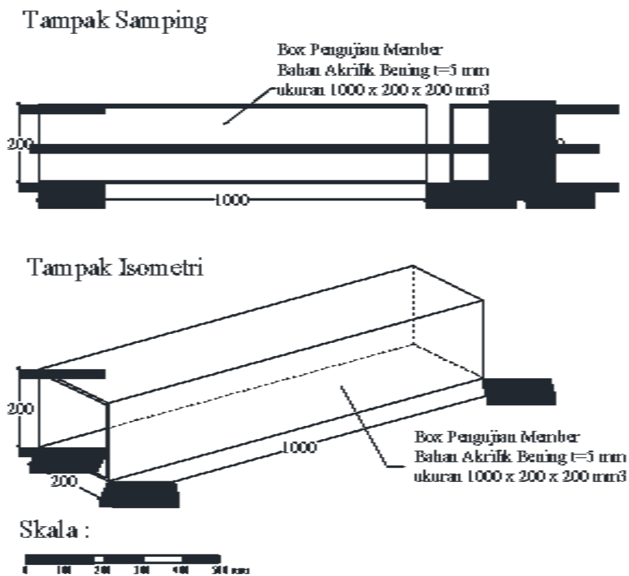
Gambar 20. Abutmen untuk Pengujian Jembatan Boks Pengujian Member (satuan : mm)
