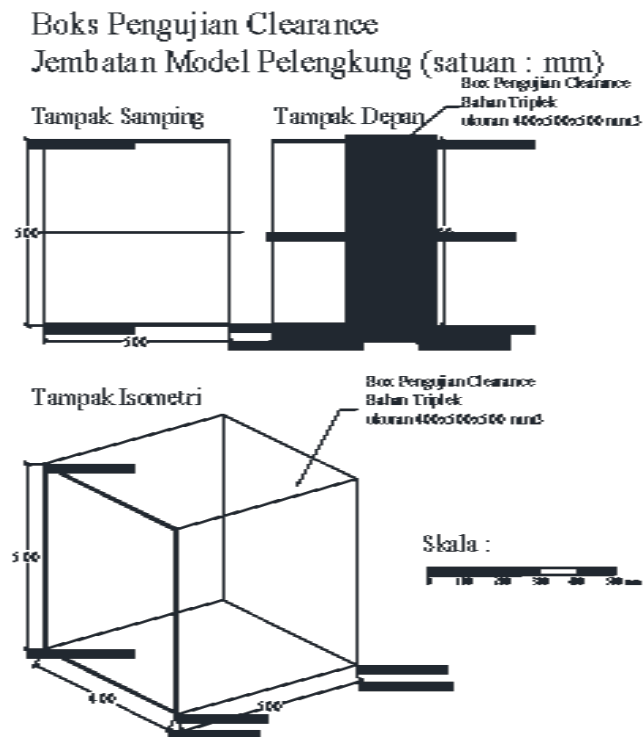
Gambar 24 Boks Pengujian Clearance Jembatan Model Pelengkung
