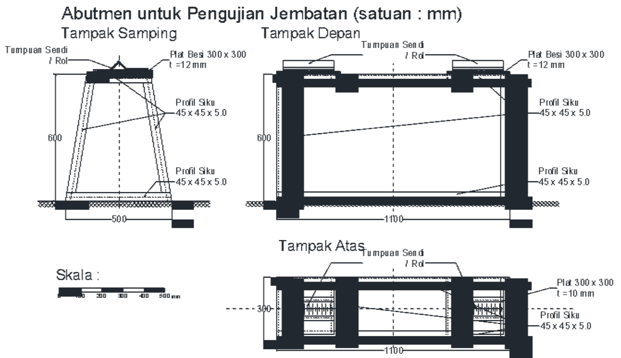
Gambar 7. Abutmen Untuk Pengujian Jembatan
